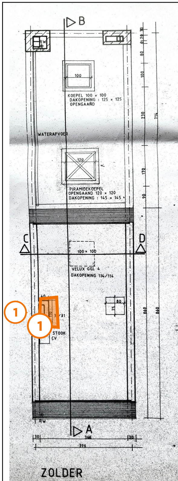
Legende van plan 1.3: Brander ACV
