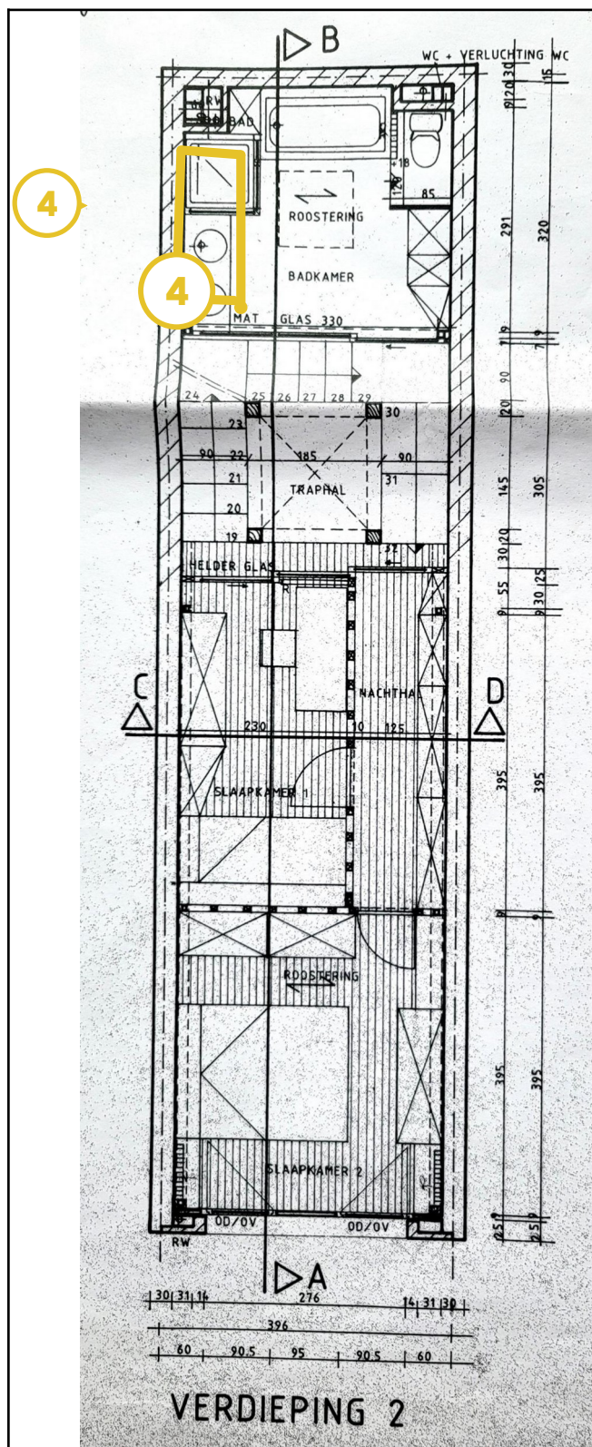
Legende van plan 1.10: VERDIEPING 2 - badkamermeubel
