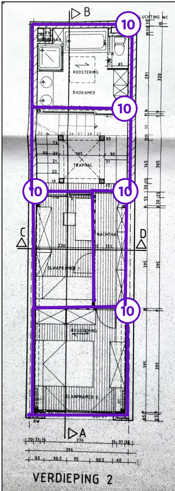
Legende van plan 1.6: VERDIEPING 2 - binnenwanden
